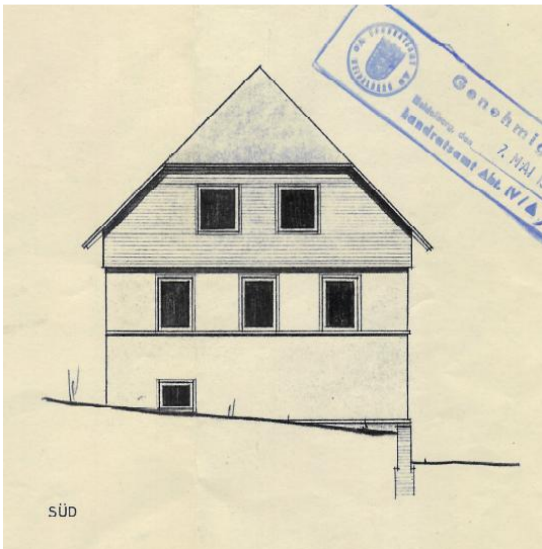
Ansicht Süd:
